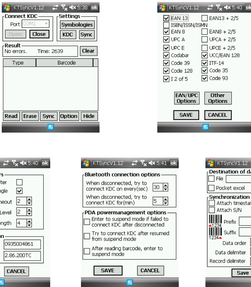
図 31- Mobile pKTSync
