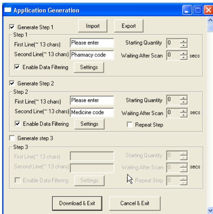
図 37-Application Generation Menu
