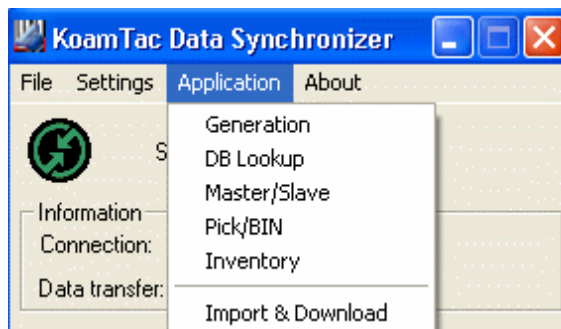
図 22- Application Menu
