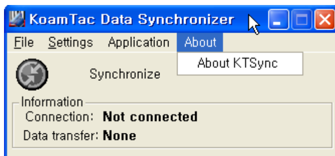
図 23-About Menu
