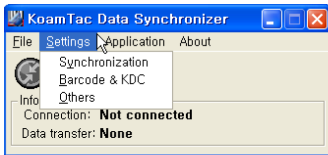
図 21 - Setting Menu
