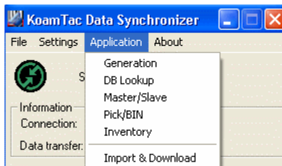
図 35-Application Menu
