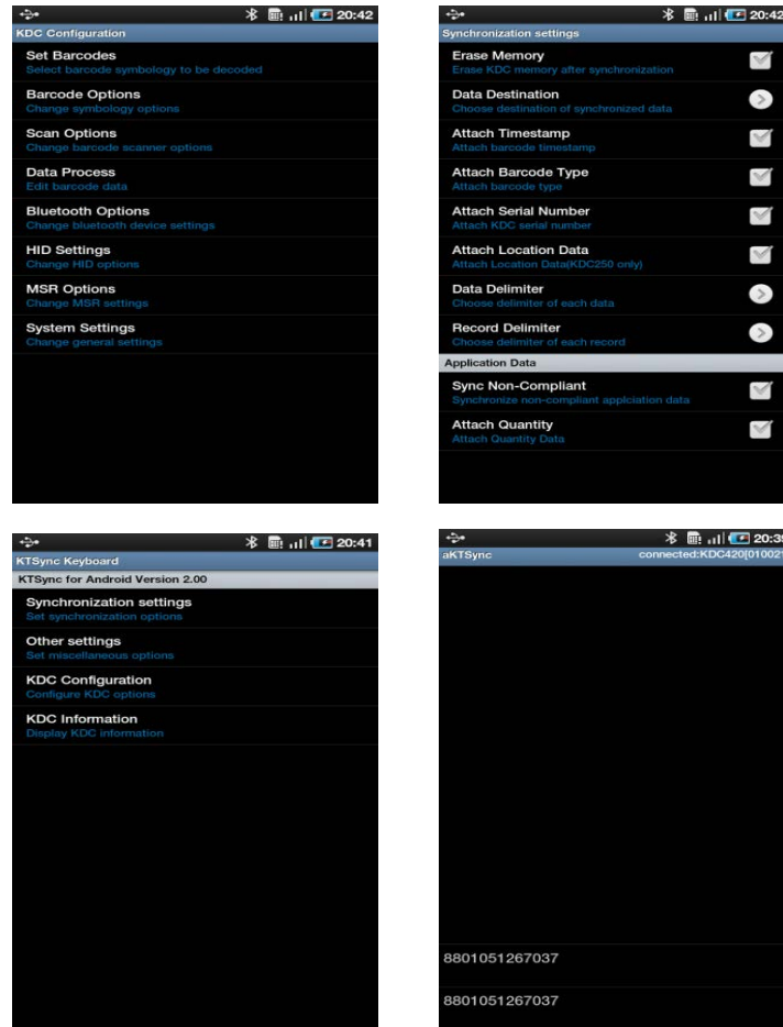
図 32-Android aKTSync
