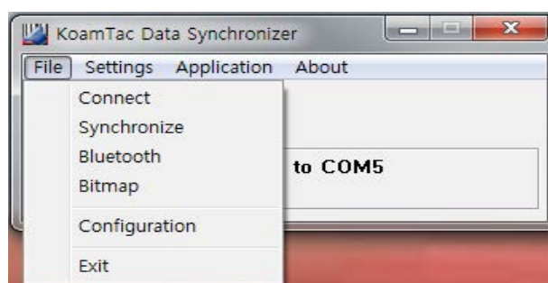
図 20-File Menu
